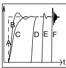
Fig.: 控制器的阶跃响应
