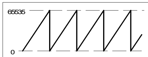
Fig.: 正相旋转的脉冲编码计数器的曲线形状。
